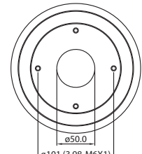
vista inferior
