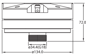
vista lateral
